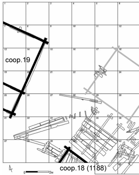
Рис. 5. Усадьба Нкл2007-III. Схема застройки
