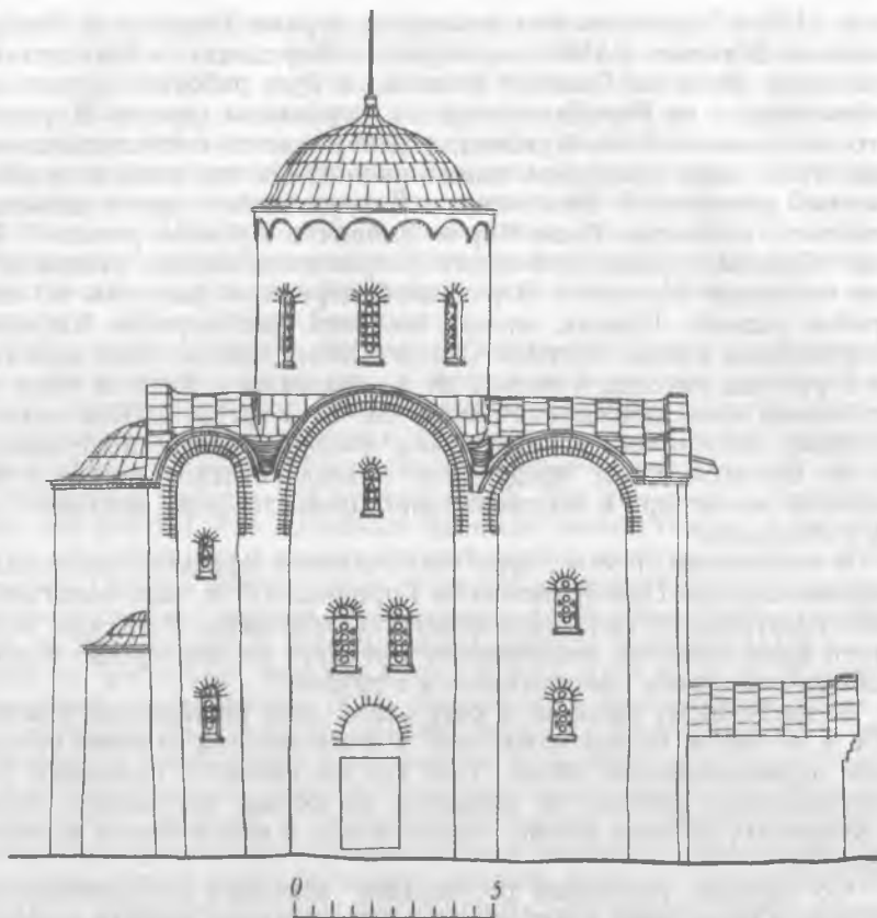
Рис. 1. Реконструкция первоначального облика церкви Спаса на Нередице. Г. М. Штендер. 1986 г. Северный фасад. Чертеж Л. Корчагиной.
