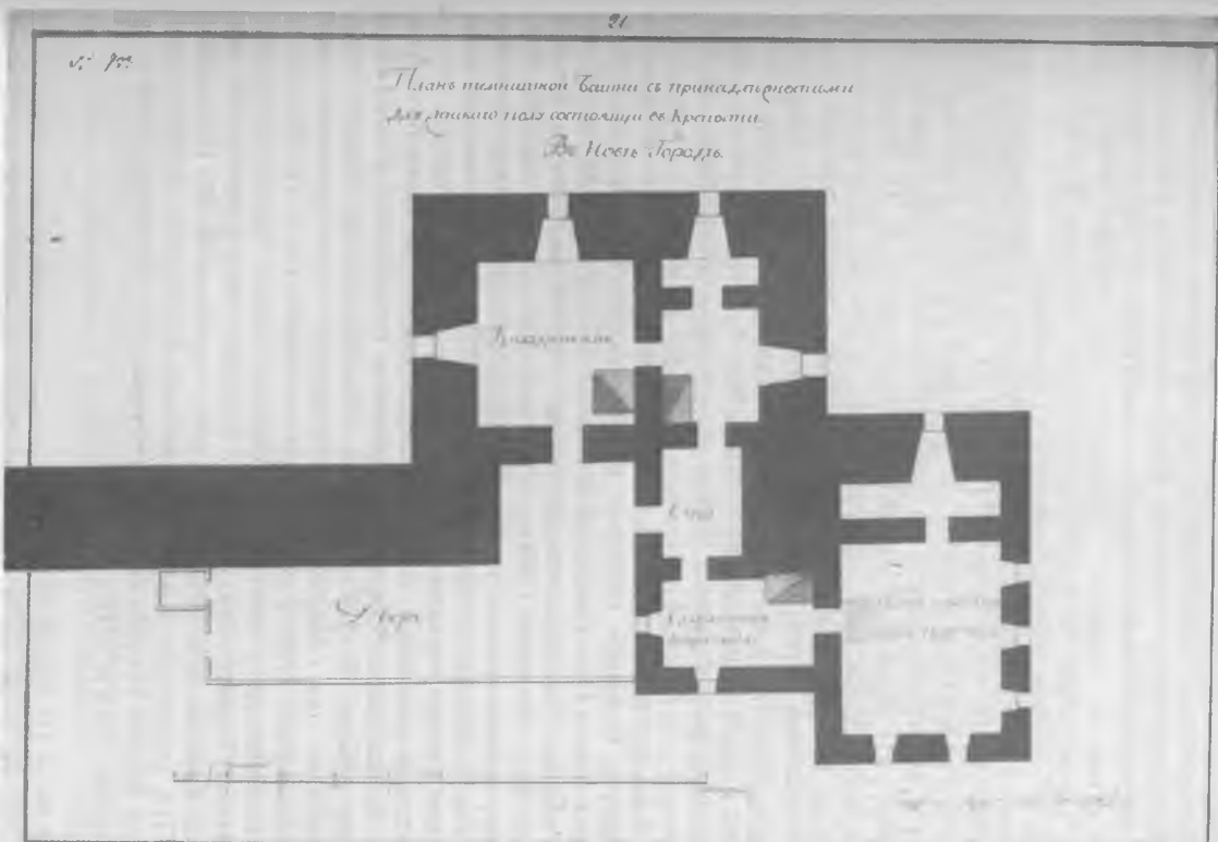
Рис. 2. Чертеж приспособленной под женскую тюрьму Покровской башни И. Дмитрова. 1816 г.
