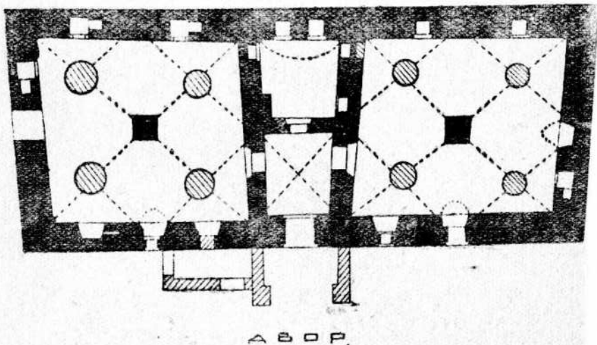
Рис. 1. Дом купцов Русиновых XVII века во Пскове, ул. Карла Маркса, № 10.
