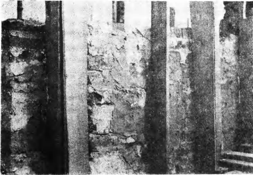
Рис. 14. Северная лопатка западного фасада Нередицкой церкви. Возведение кладки по маякам-шаблонам.
