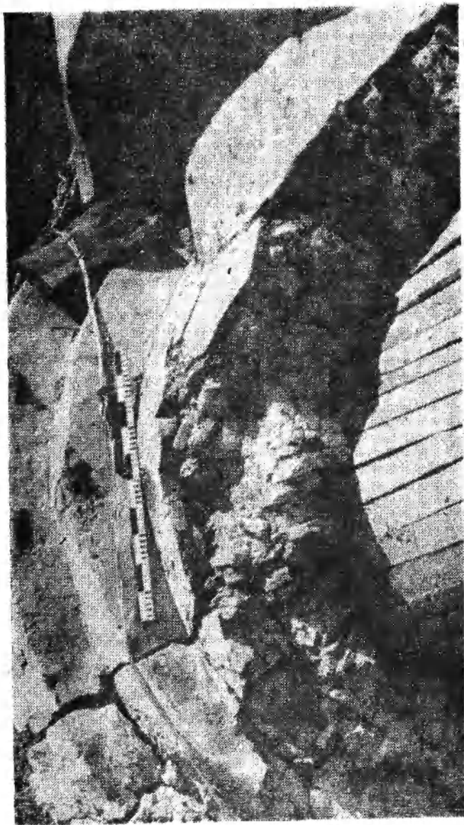
Рис. 11. Фрагмент юго-восточного свода Перелик зі перкви (контра-столи в дна переката).
