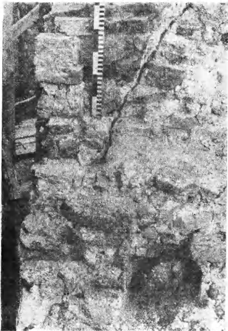
Рис. 4. Верхняя часть кладки центральной апсиды Неридицкой церкви. Вид с севера. (Слева видна позднейшая надкладка стены).
