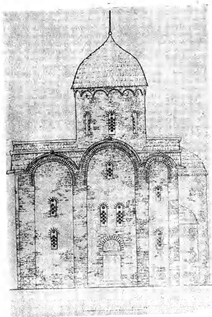
Рис. 12. Древний облик Нередицкой церкви. Реконструкция автора
